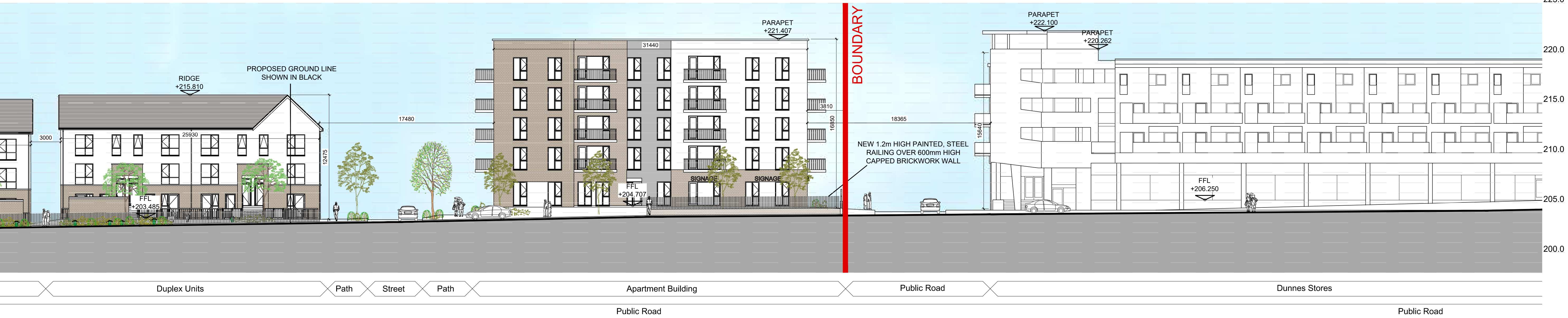
SITE SECTION A-A (PART B) SCALE 1:200@A1
