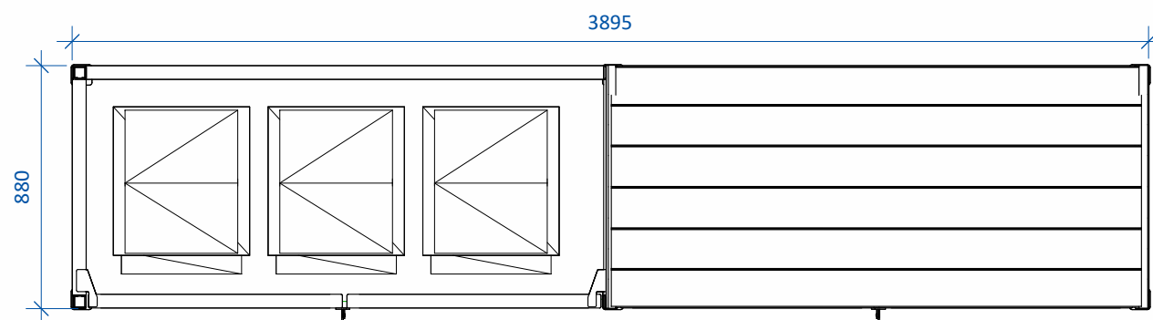
Roof Plan; 1:25
